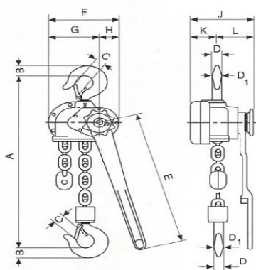
Pullift D95 1.500-3.000 kg
