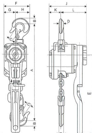
Type AL 750-3.000 kg
