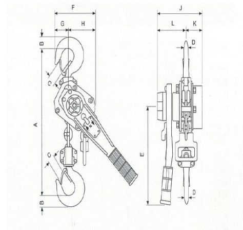
Type PT 750-6.000 kg
